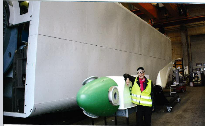
Annelise Laursen har vært ansatt hos Bonus/Siemens i 28 år. Nacellen på 30 kW-mallen som er vist her veier kun 1,645 kg. Til sammenligning veier 3,6 MW nacellen 125 tons.
